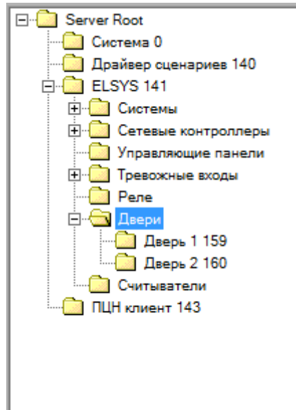
Рис. 4. Дерево тегов OPC-сервера в режиме «По типам устройств»
